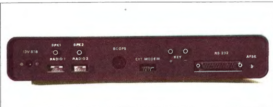
Tyłna ścianka — wejścia i wyjścia modemu
