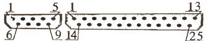
Rys. 2. Sygnały złącza RS232
