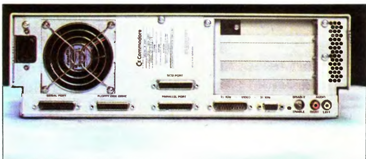
Tylna ściana obudowy — komplet złącz
