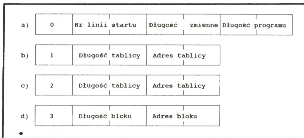
Rys. 3 Struktura nagłówek plików: a) program w języku BASIC, b) tablica liczbowa, c) tablica znakowa, d) typ CODE.
