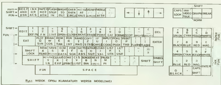
Rys. 4 WIDOK OPISU KLAWIATURY WERSII MODELOWEJ
