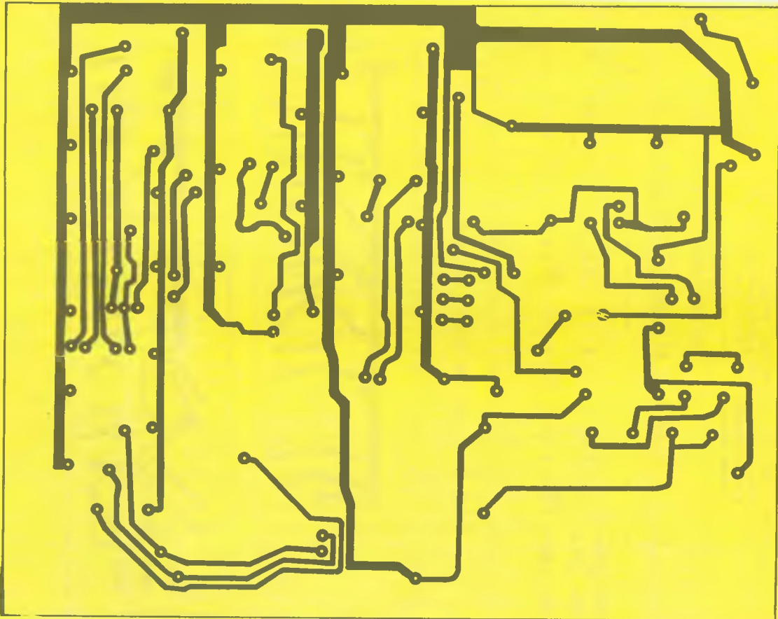
rys.3.c. PŁYTKA DRUKOWANA -STRONA ELEMENTÓW (WIDOK OD STRONY ELEMENTÓW)
