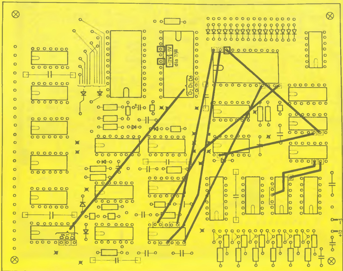
Rys. 1d PŁYTKA DRUKOWANA – WIDOK OD STRONY LUTOWANIA – POŁĄCZENIA PRZEWODEM [CYNĄ]
