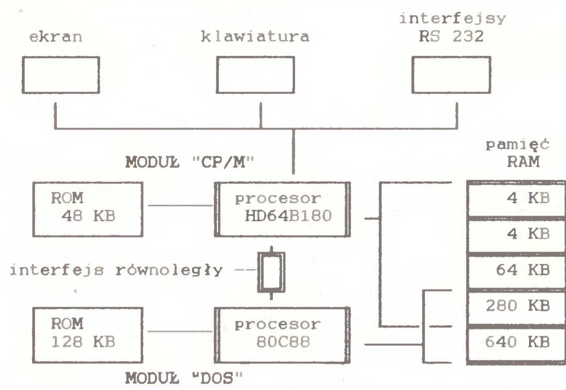
Rys. Schemat budowy wewnętrznej i sposób wykorzystania pamięci RAM komputera Husky Hawk 8/16.
