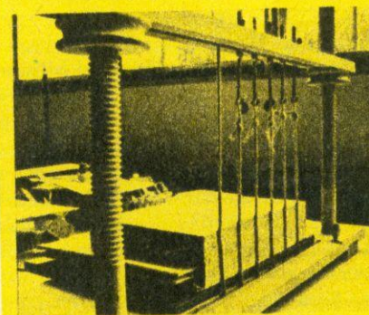
Prace introligatorskie – łączenie poszczególnych akładek
