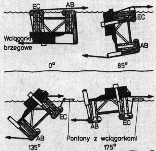
Etapy odwracania platformy „Alexander L. Klelland”
