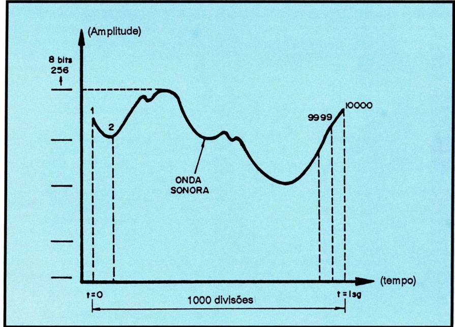
Representação de um sinal sonoro com 8 bits de amplitude e 10 000 impulsos por segundo
