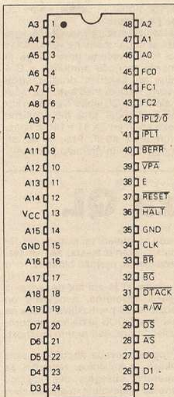
Razpored nogic mikroprocesorja MC 68008
