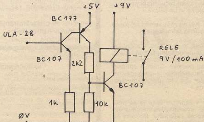
Skica 3: nadzor nad motorjem kasetofona
