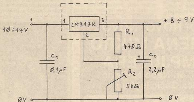
Skica 1: stabilizator napetosti
